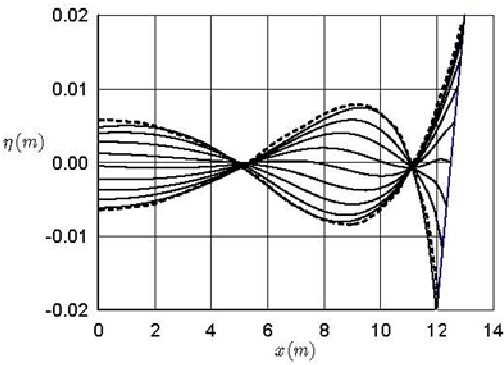
圖 1 波浪傳遞於斜坡底床之波浪溯升
